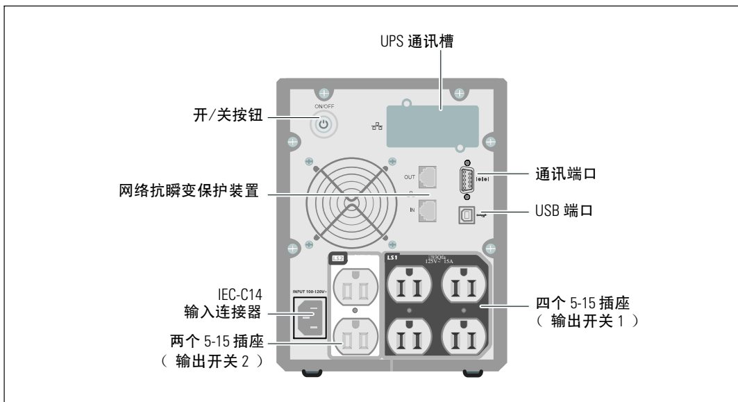
图 3. 500W，100/120V 后面板
